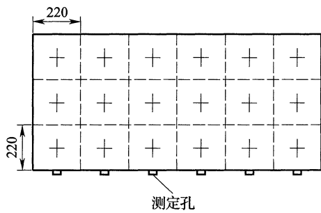
图 E. 1. 3-1 矩形风管测点布置示意
