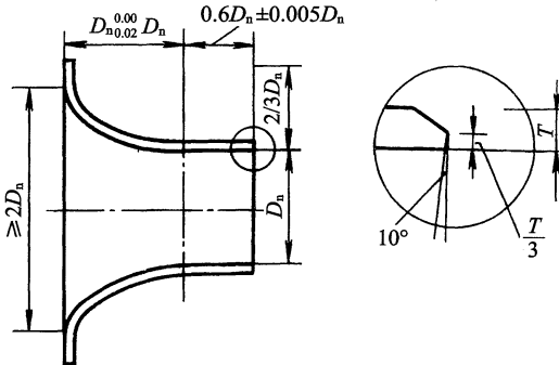
图 C.2.7-2 标准长颈喷嘴
