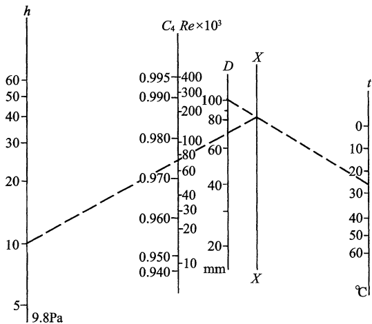
图 C. 2. 7-3 喷嘴流量系数推算图
