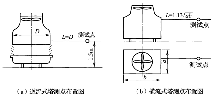
图 E. 6. 1-1 冷却塔测点布置图
