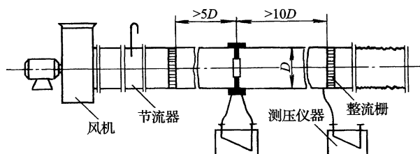
图 C. 2. 6-3 负压风管式漏风量测试装置
