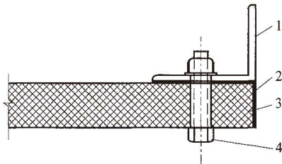
图 4.3.3 玻璃纤维复合风管角钢连接示意
