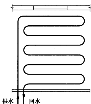
图 3 平行型布置
