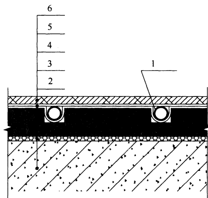
图 A.0.2-1 与供暖房间相邻的预制沟槽保温板式供暖地面构造
